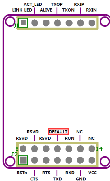
图 2-2 W5500S2E-S1 模块管脚图
