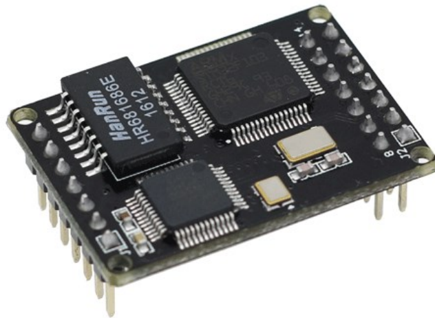
图 2-1 W5500S2E-S1 模块外形图
