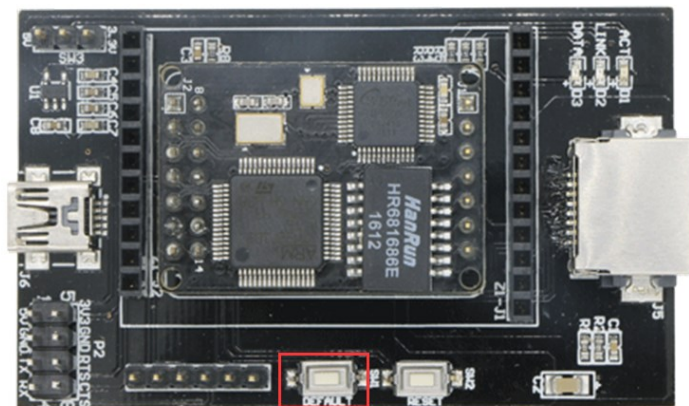
图 5-3 通过评估板恢复出厂设置
