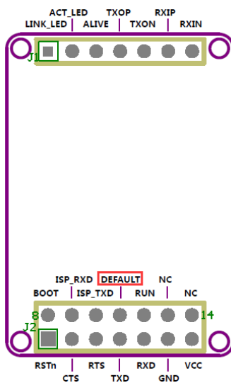
图 5-4 通过模块 DEFAULT 管脚恢复出厂设置
