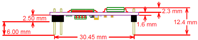
图 1-2 W5500S2E-S1 模块机械尺寸图-侧视图
