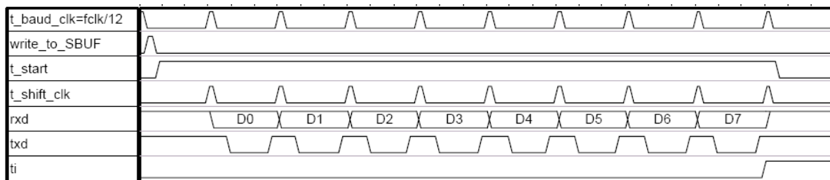
Fig. 9-1: TranOBit mode 0
