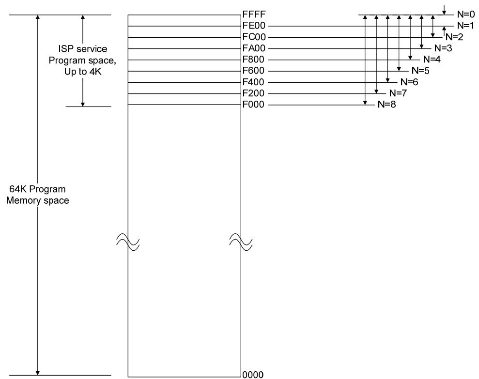
Fig. 3-1: SM5964B programmable Flash
