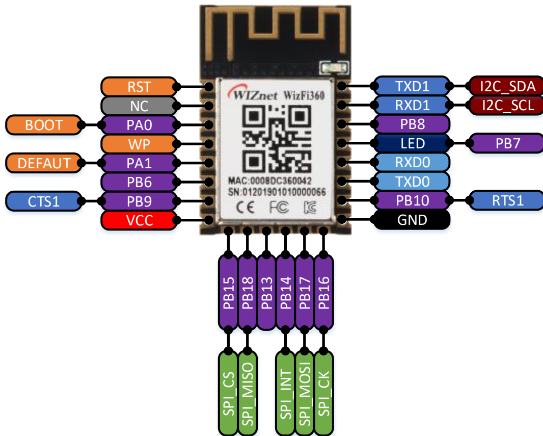
Figure 3. WizFi360 Pinout
